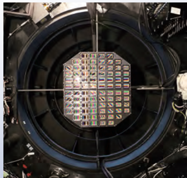
シュミット望遠鏡の焦点部に設置された Tomo-e Gozen カメラ
